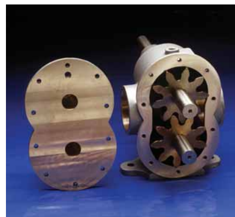
Deltapumpen, enkel og robust konstruksjon.
